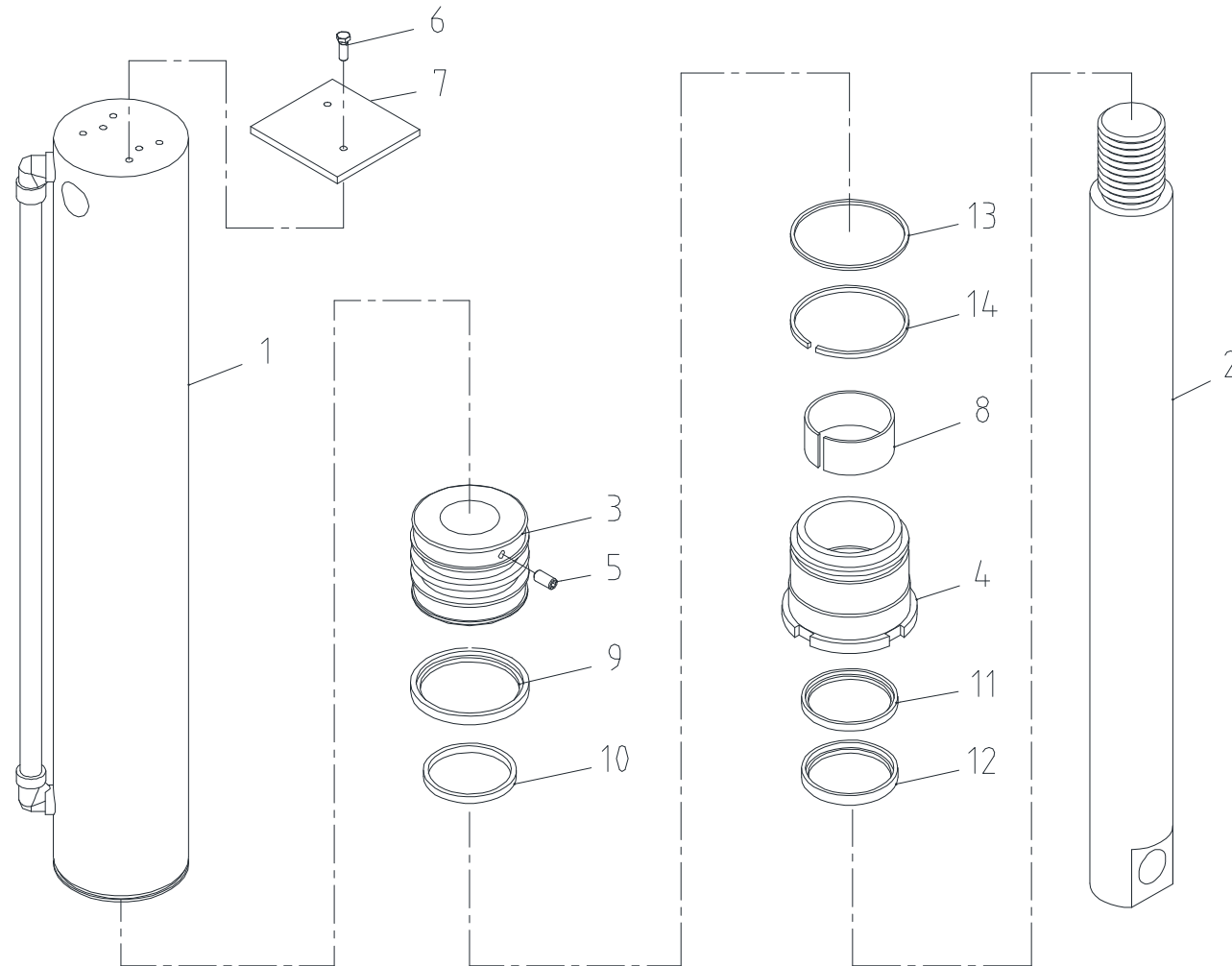
잭 실린더 조립체 Fig. 9-2-1-1 SCS1216 JACK CYL' ASS'Y
