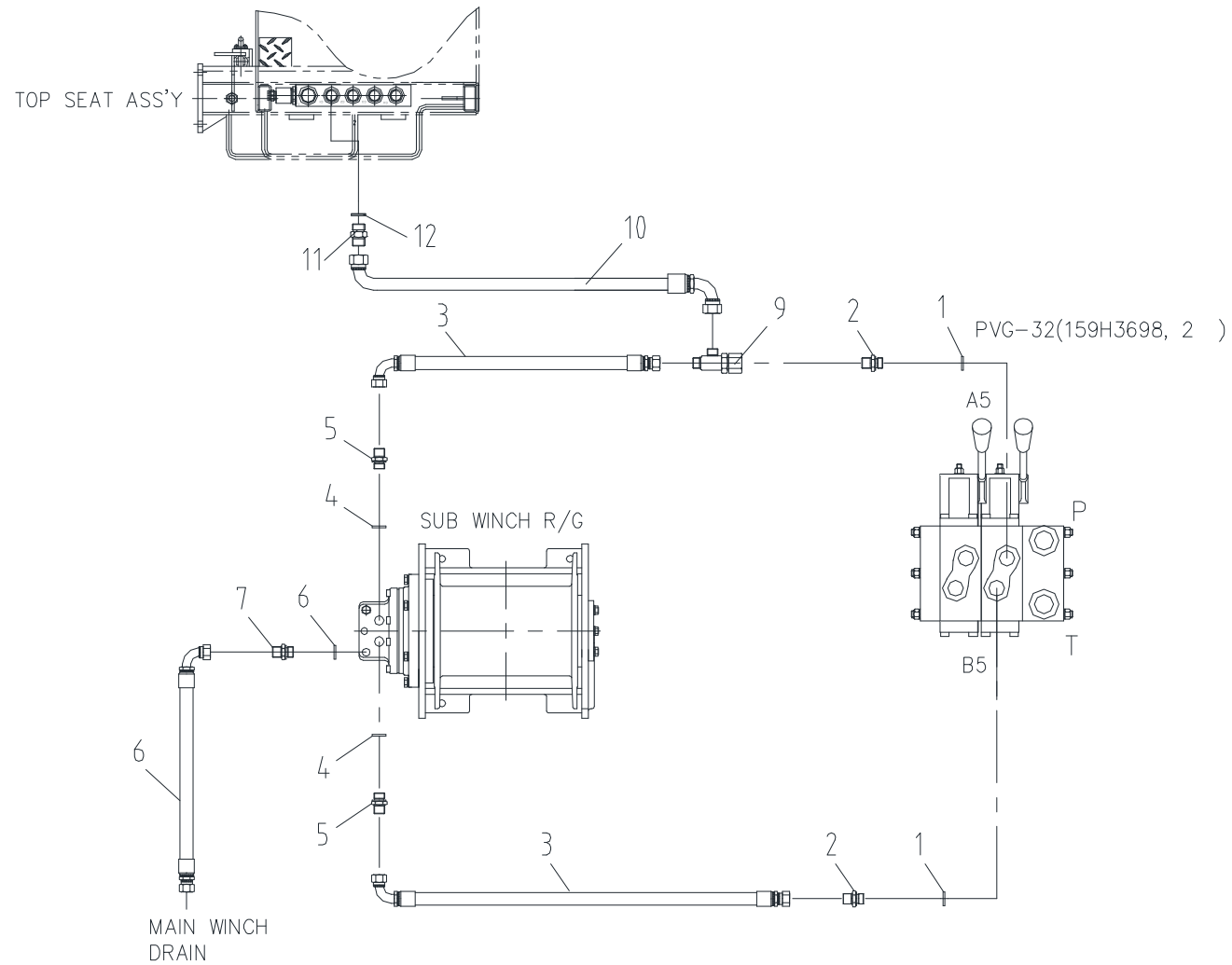
보조 원치 배관 Fig. 13 SUB WINCH PIPING
