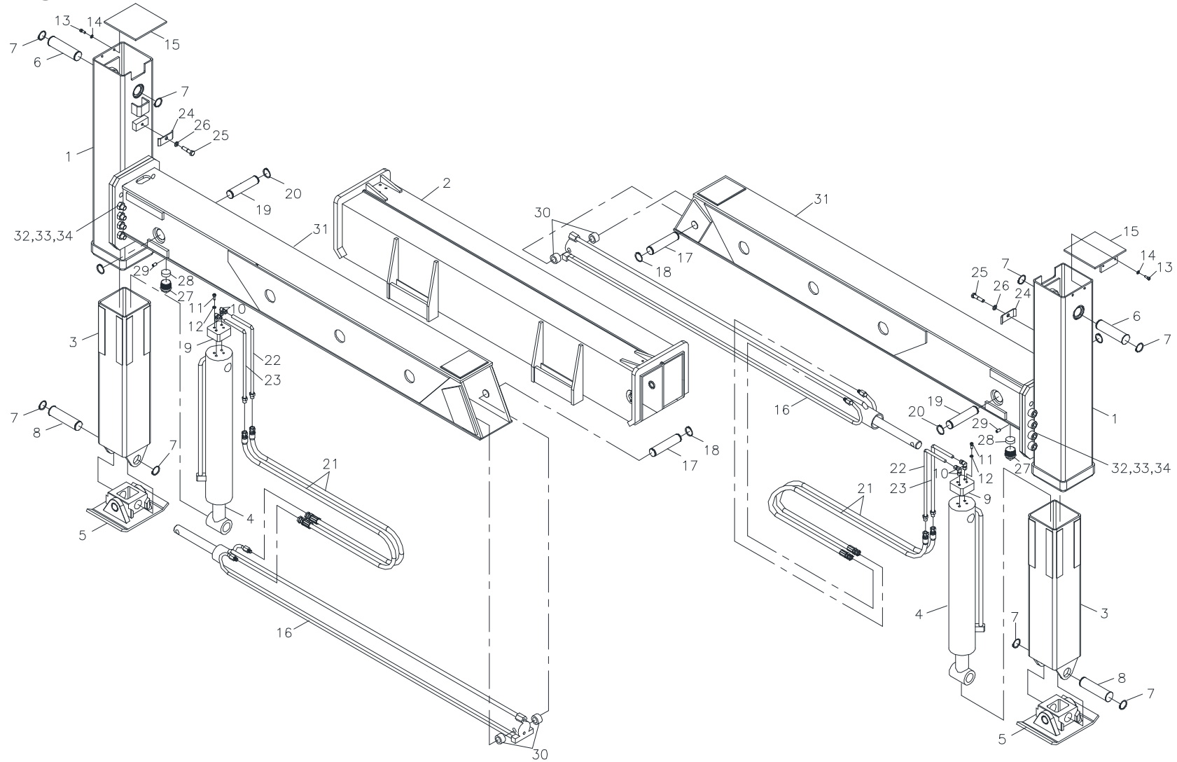
후방 아웃리거 조립체 Fig. 9-2-1 SCS1216 REAR OUTRIGGER ASS'Y
