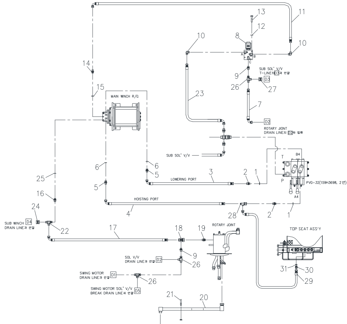
메인 윈치 배관 Fig. 5-5 SCS1216 MAIN WINCH PIPING
