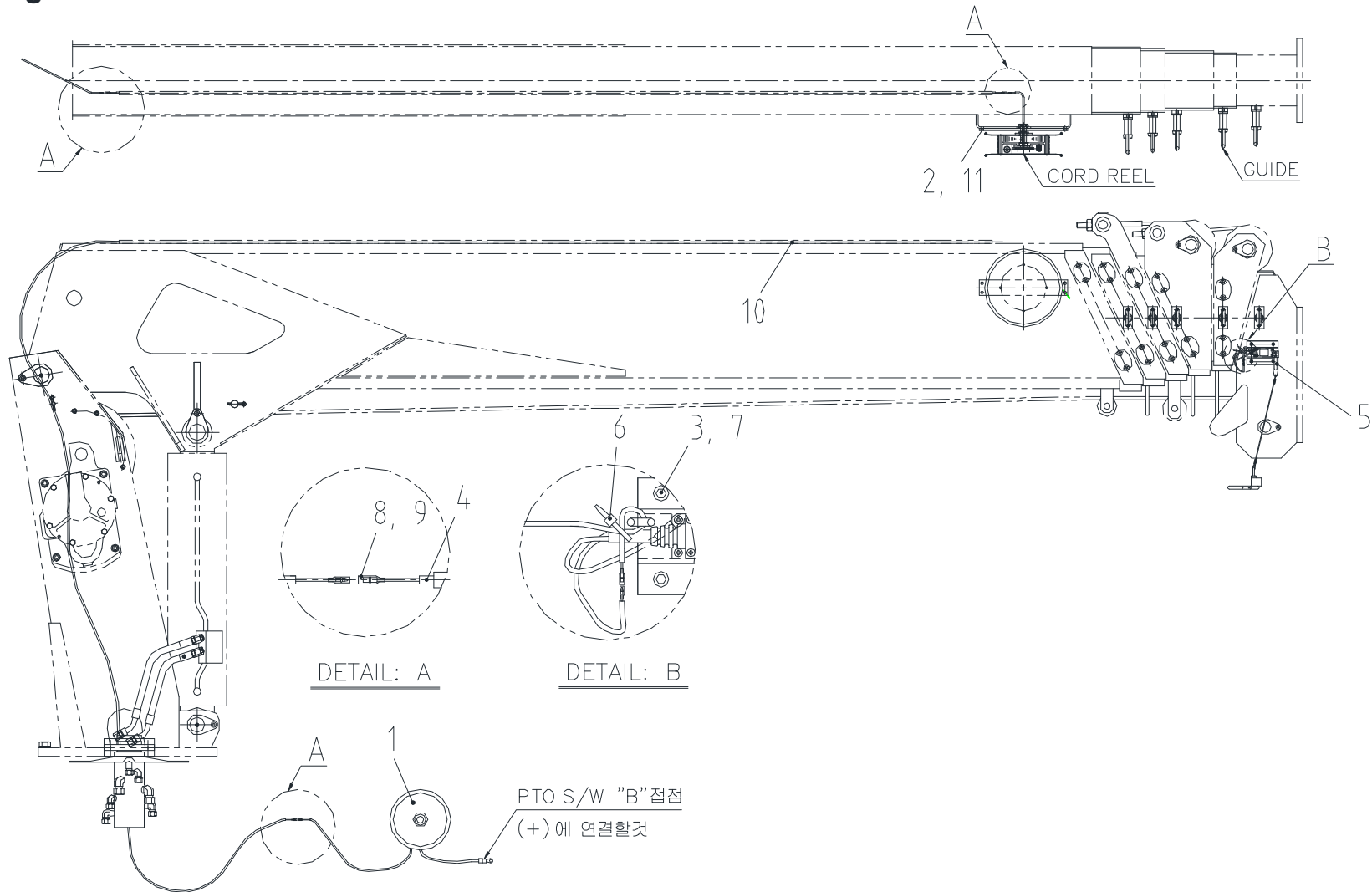
Fig. 14 과권방지장치 조립체
