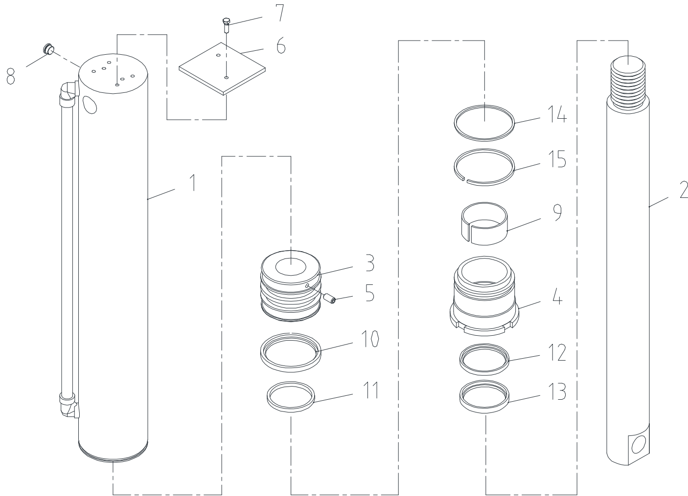
잭 실린더 조립체 Fig. 4-2 SCS1216 JACK CYL' ASS'Y
