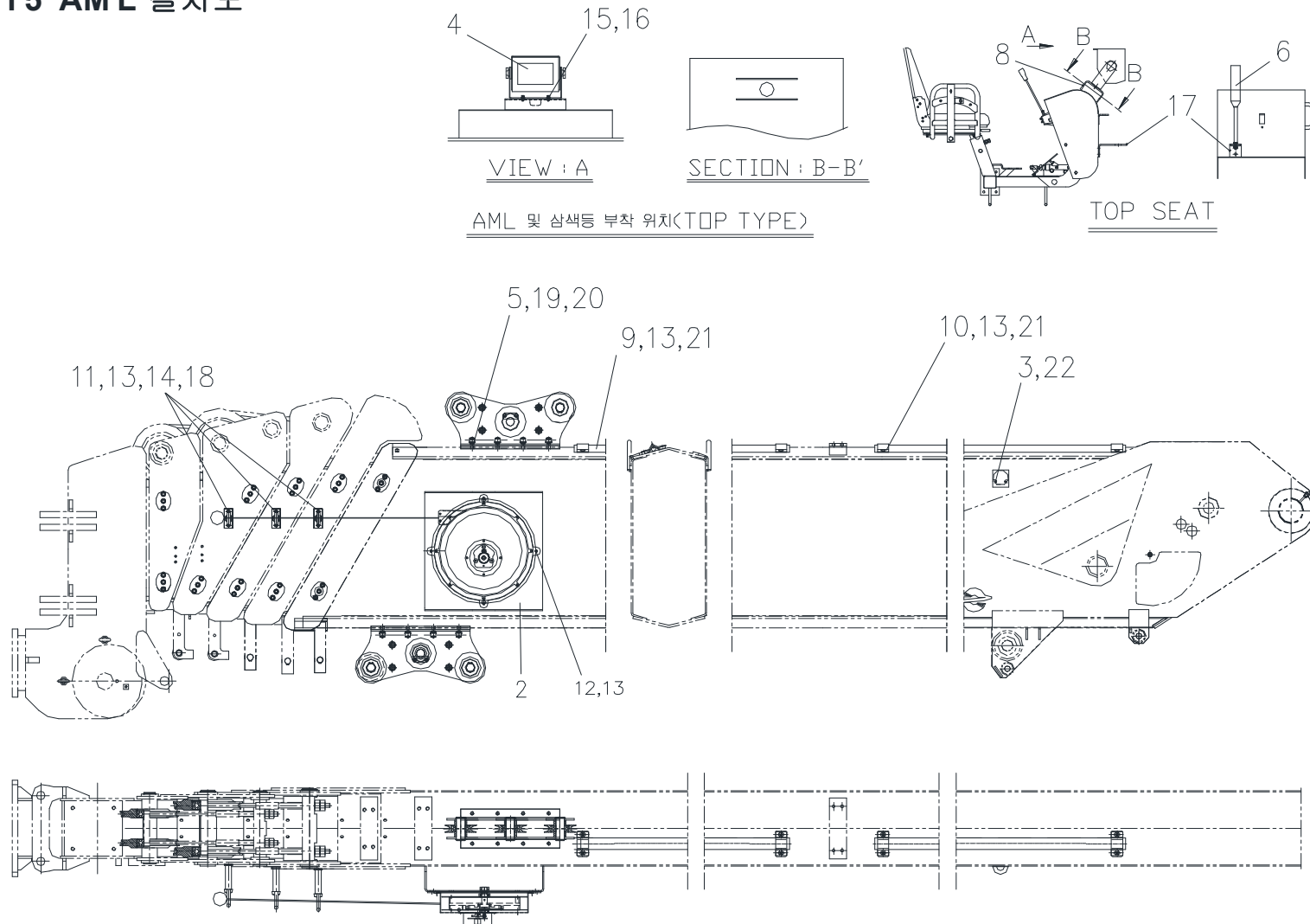
Fig. 15 AML 설치도
