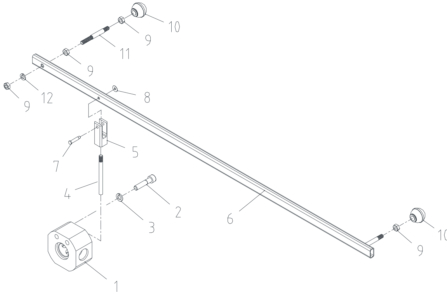
디버터 밸브 셋 Fig. 3-3 SCS1216 DIVERTER V/ V SET
