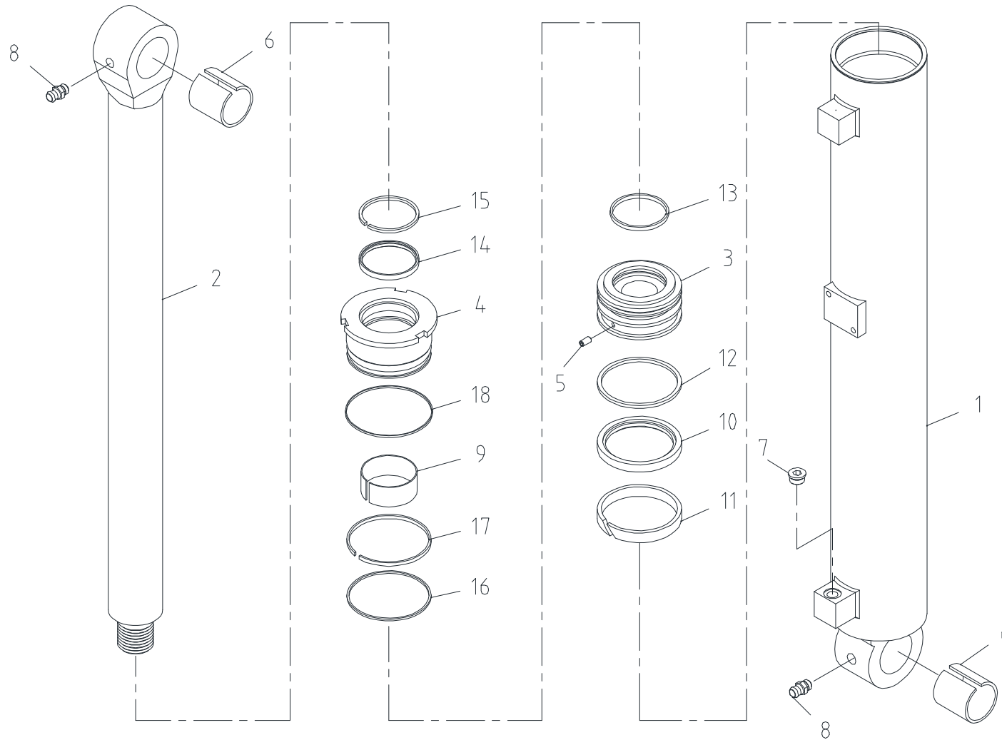
데릭 실린더 조립체 Fig. 2-2 SCS1216 DERRICK CYL' ASS'Y
