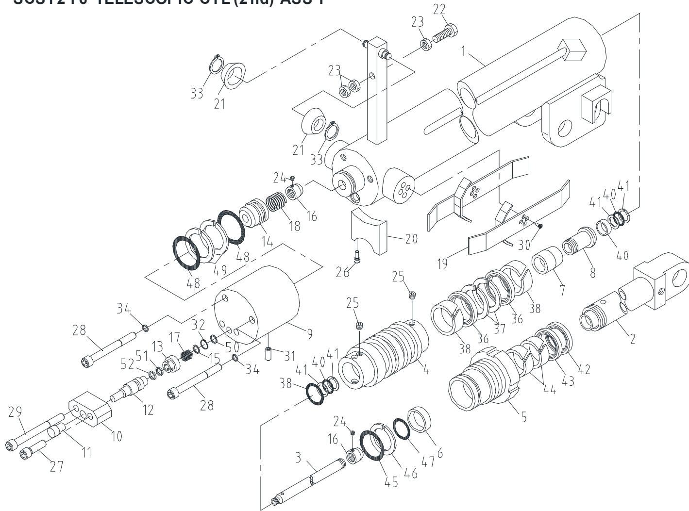
텔레스코픽 실린더(2단) 조립체 Fig. 1-1-2 SCS1216 TELESCOPIC CYL'(2nd) ASS'Y
