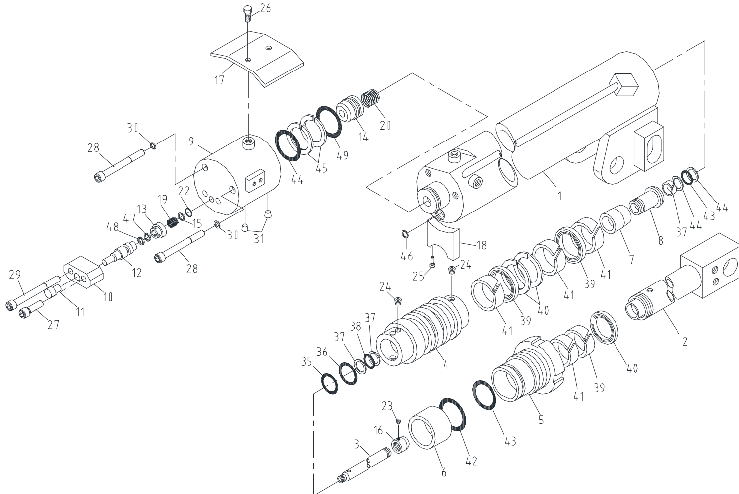
텔레스코픽 실린더(1단) 조립체 Fig. 1-1-1 SCS1216 TELESCOPIC CYL'(1st) ASS'Y
