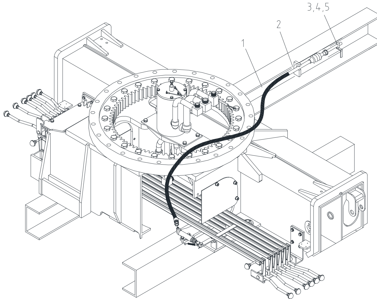
악셀 시스템 파트 Fig. 9-3 SCS1216 ACC'L SYSTEM PART
