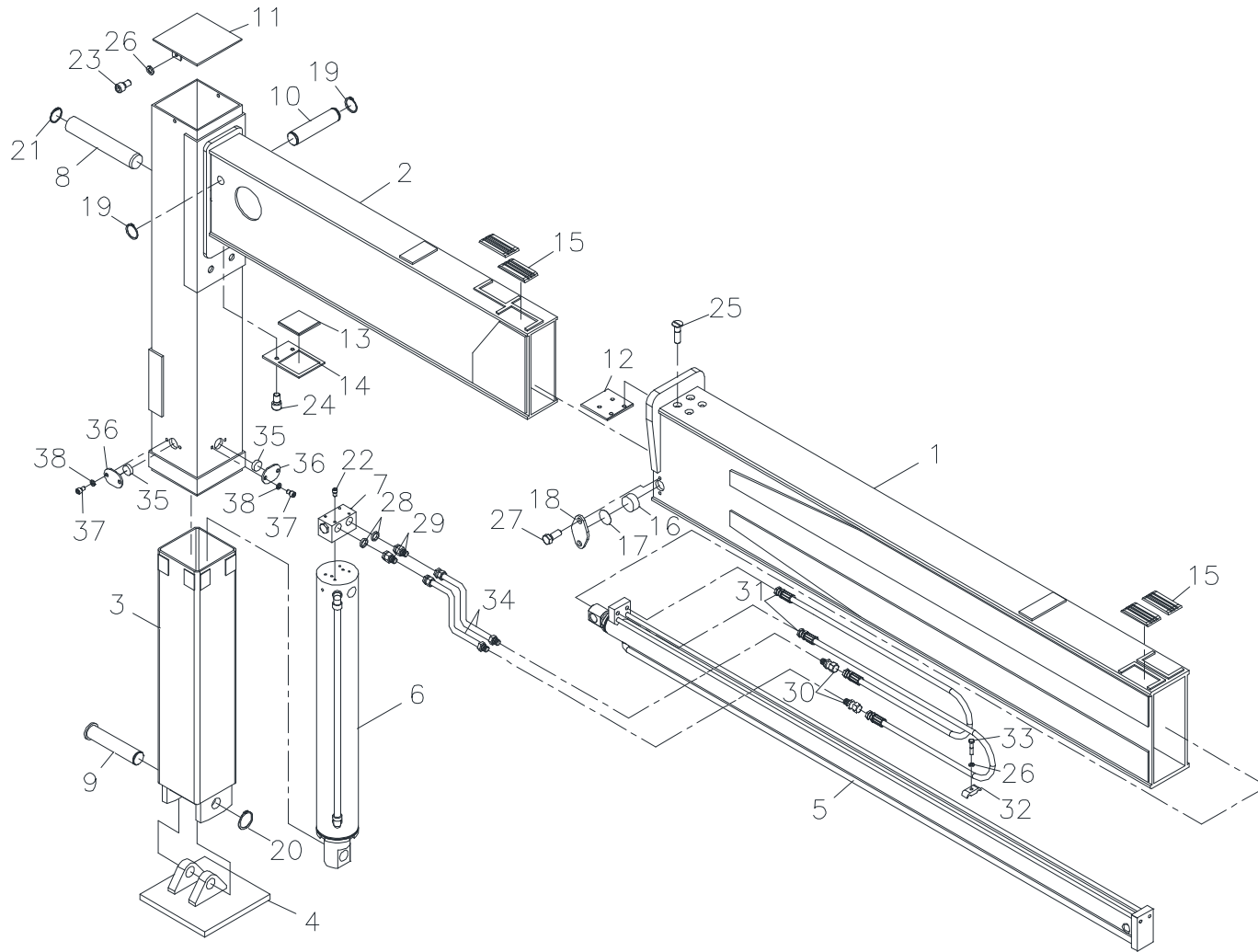
아우트리거 조립체 Fig. 4 SCS1216 OUTRIGGER ASS'Y
