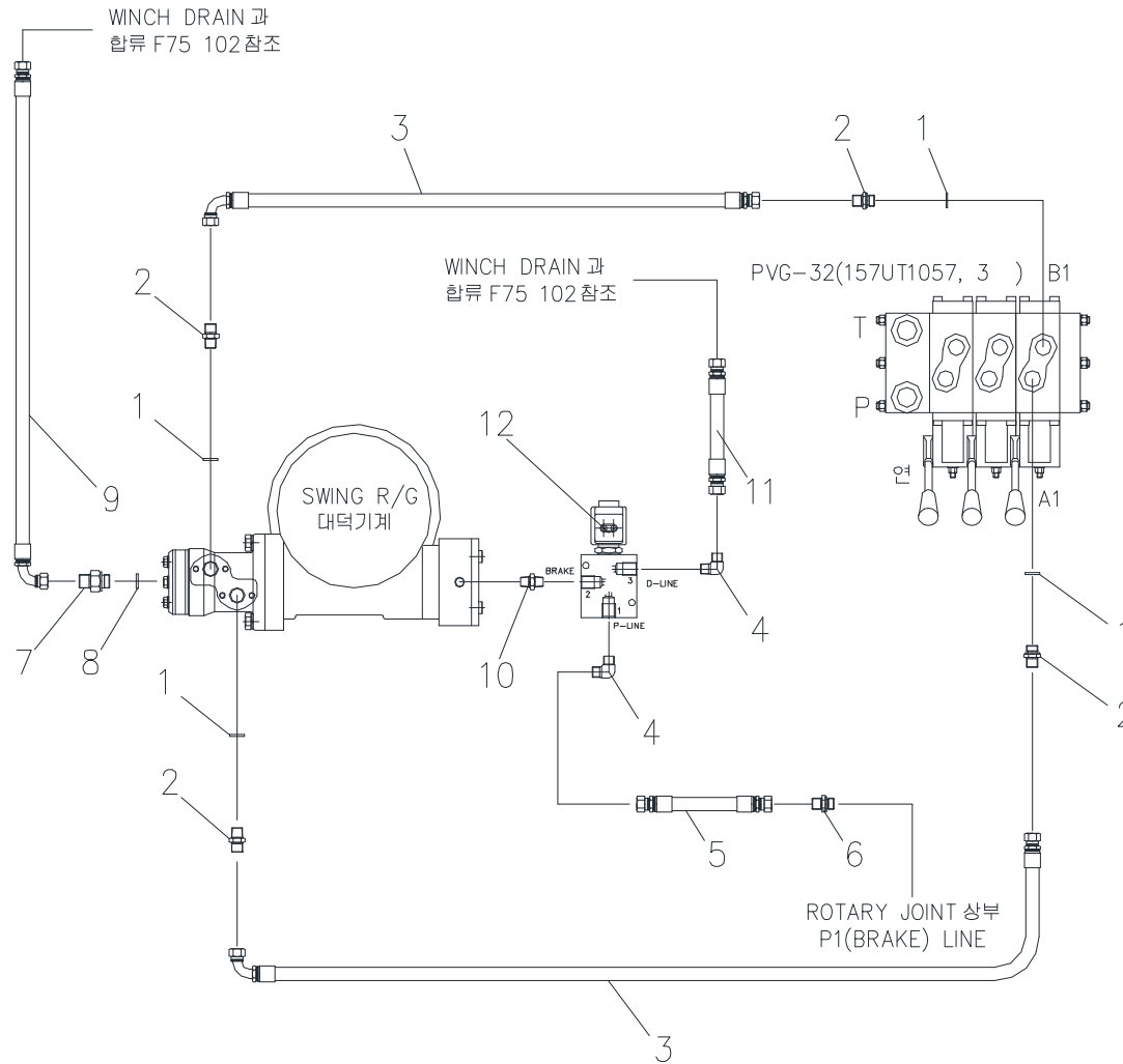
스윙 배관 Fig. 5-2 SCS1216 SWING PIPING
