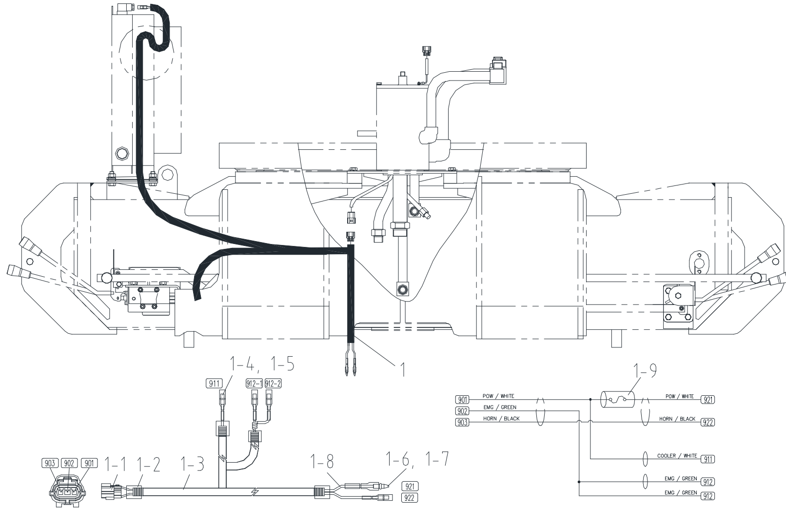
프레임 전선 Fig. 10-1. SCS1216 FRAME WIRING
