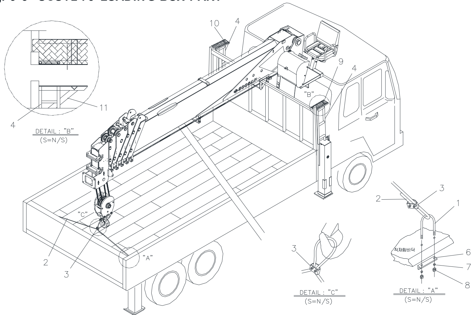
로딩 박스 파트 Fig. 9-5 SCS1216 LOADING BOX PART
