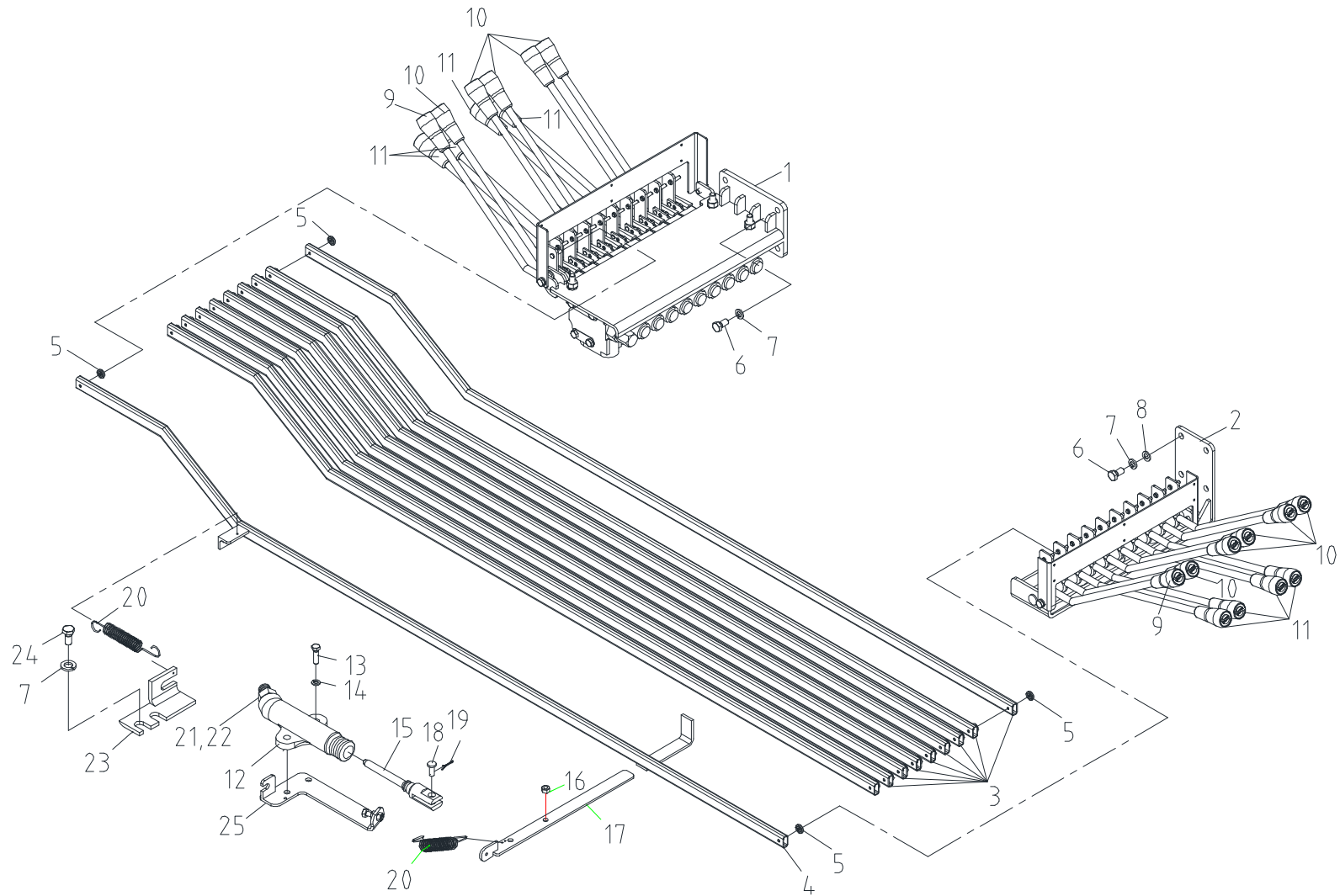
오퍼레이션 조립체 Fig. 3-2 SCS1216 OPERATION ASS'Y
